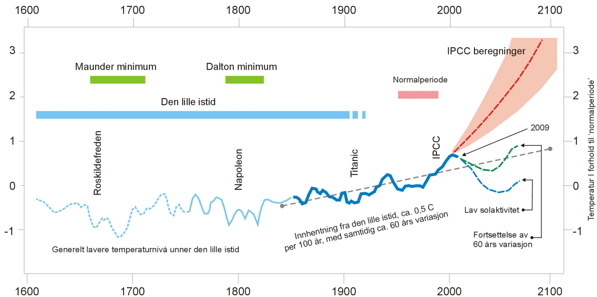
Figur som viser global temperaturutvikling fra år 1600 i forhold til normalperioden 1960-90. Kurvene viser: blå er målt temperatur siden 1850 (HadCRUT3); lyseblå er mindre nøyaktige estimater tilbake i tid; rød prikket er IPCCs prognoser; grønn er mulig temperaturutvikling av observert tendens (liten CO 2 innflytelse); blå prikket er prognose for lav solaktivitet. Grønne blokker er perioder med lav solaktivitet.
