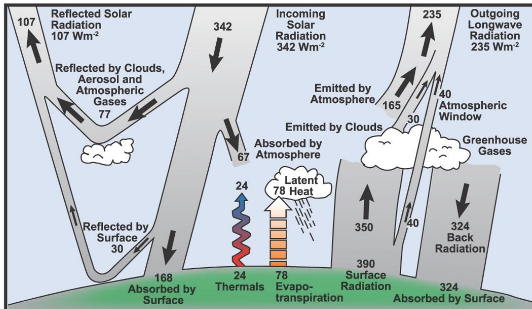
Fig. 1. Flat-jord-kald-sol-modell fra http://www.ipcc.ch/graphics/ar4-wg1/jpg/faq-1-1-fig-1.jpg
